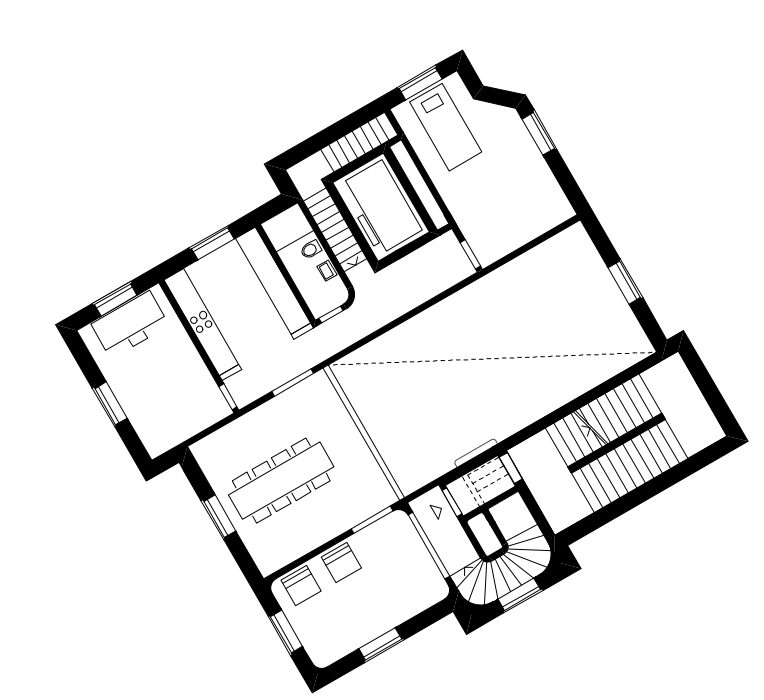
Wohnung Typ B 1: 200 Oben
