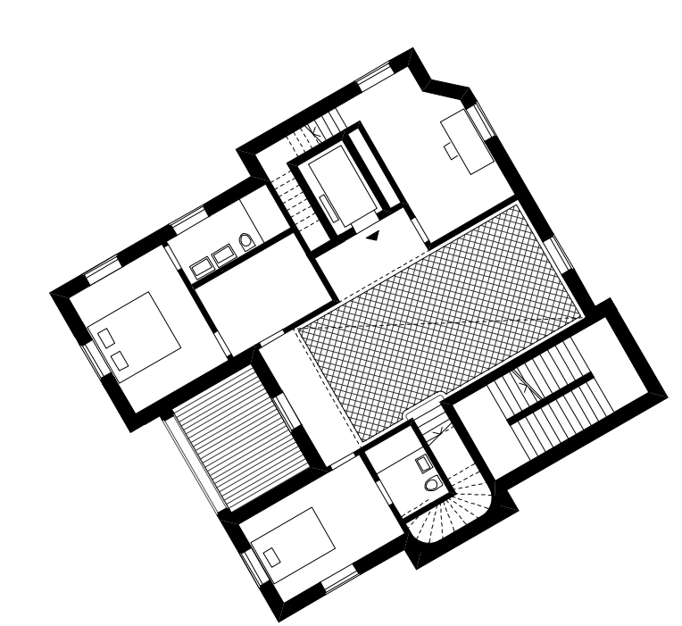
Wohnung Typ B 1: 200 Unten
