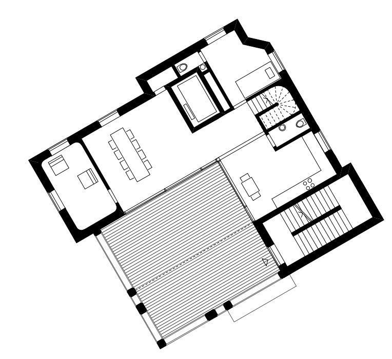
Wohnung Typ A 1: 200 Unten
