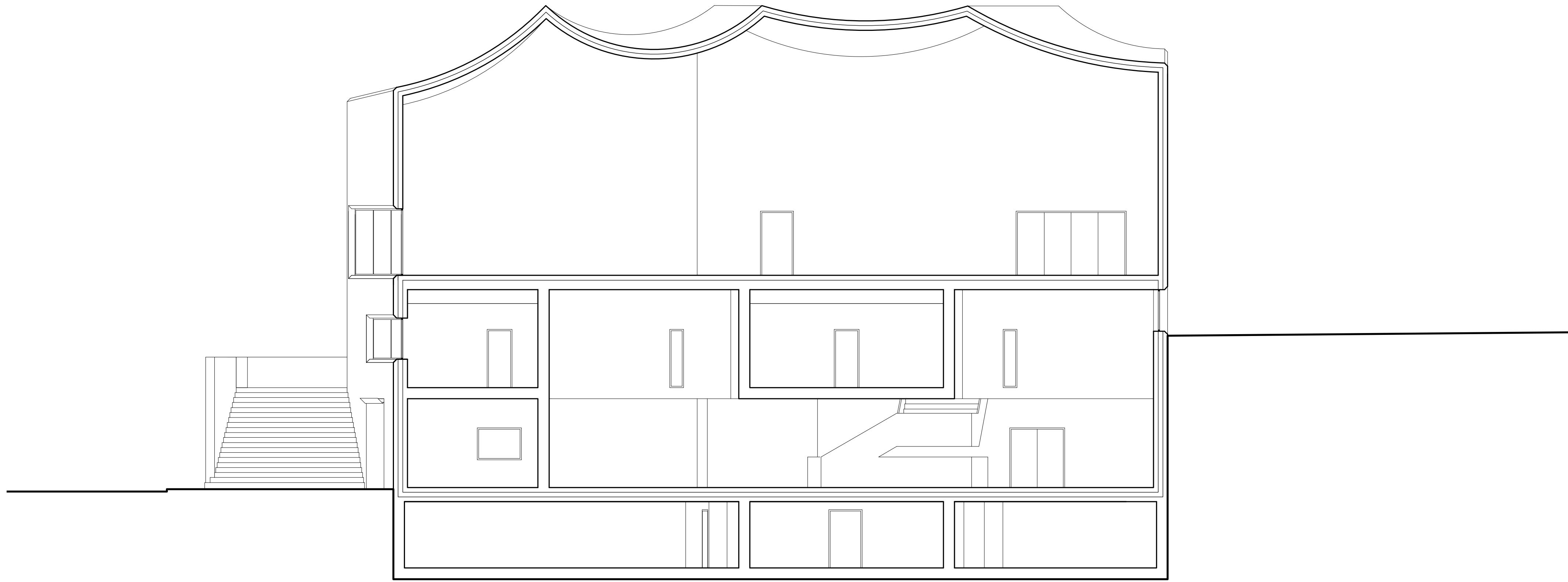
section A-A, M1:100
