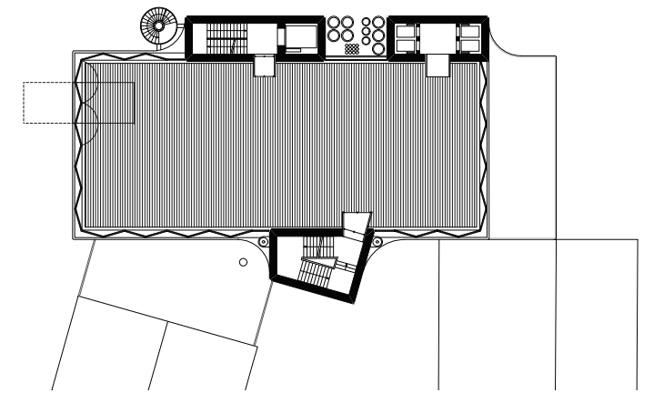
Grundriss Monatshaus M1:200
