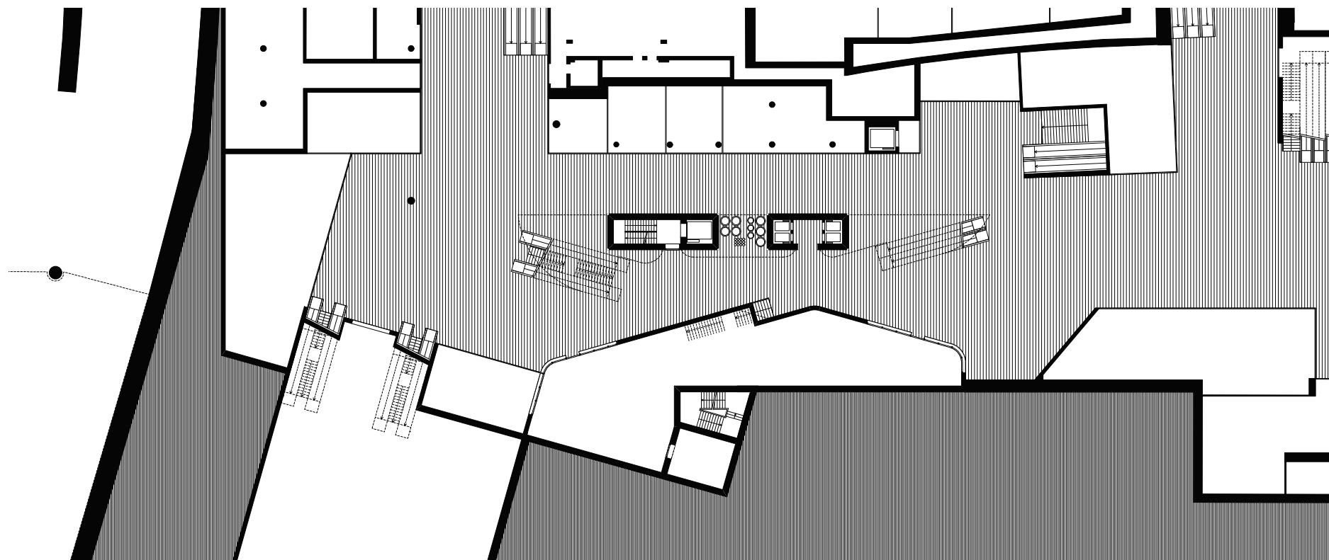
Grundriss Untergeschoss M1:200
