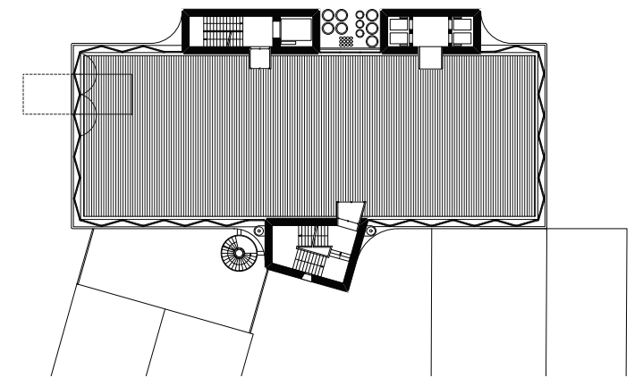
Grundriss Wochenhaus M1:200
